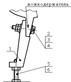
Схема №1. Крепление регулируемых ножек.
