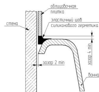
Схема №5. Установка ванны.
